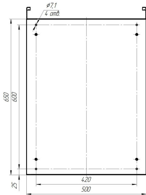
Рисунок 2 – Установочные размеры контроллера STS-504AK
