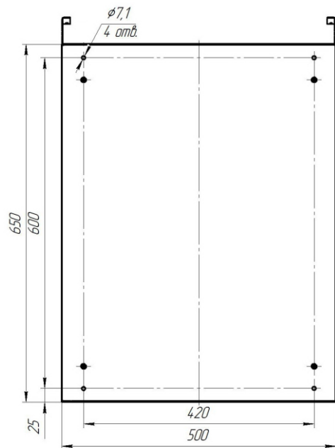
Рисунок 2 – Установочные размеры СТС-504АК
