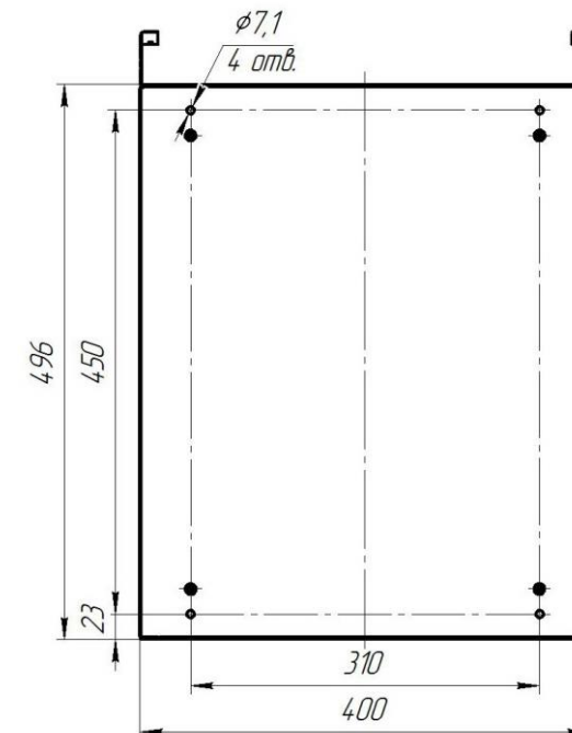
Рисунок 2 – Установочные размеры контроллера STS-504
