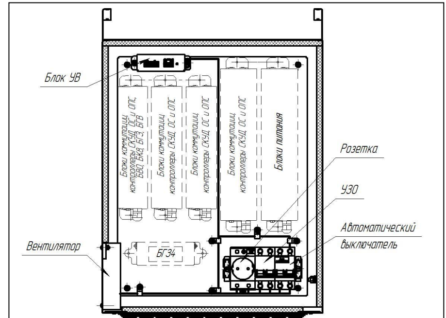
Рисунок 1 – Размещение блоков на монтажной панели
