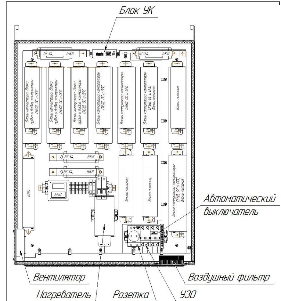
Рисунок 1 – Размещение блоков на монтажной панели (расположение элементов может отличаться от приведенного)
