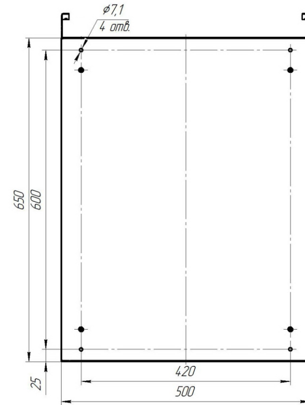
Рисунок 2 – Установочные размеры контроллера TBS-AK
