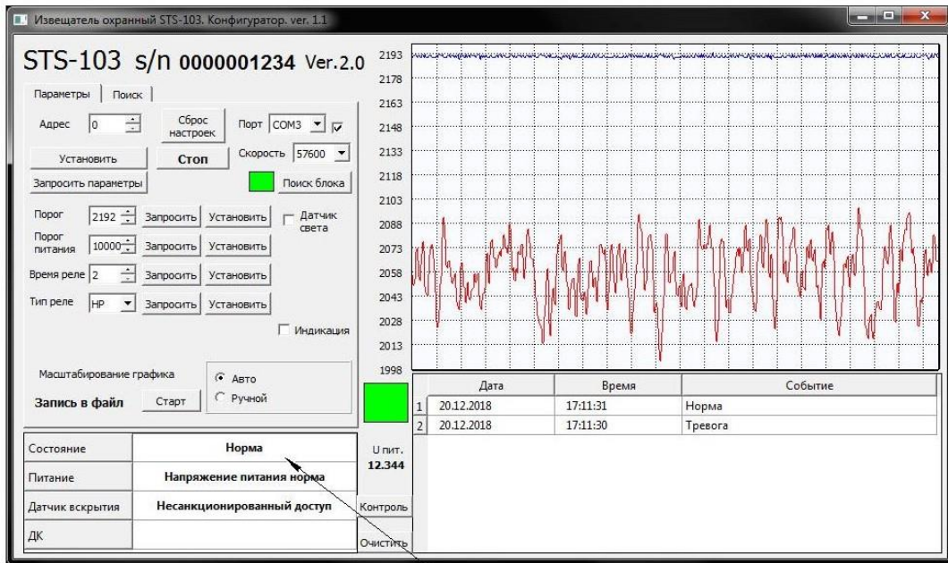
Состояние извещателя
