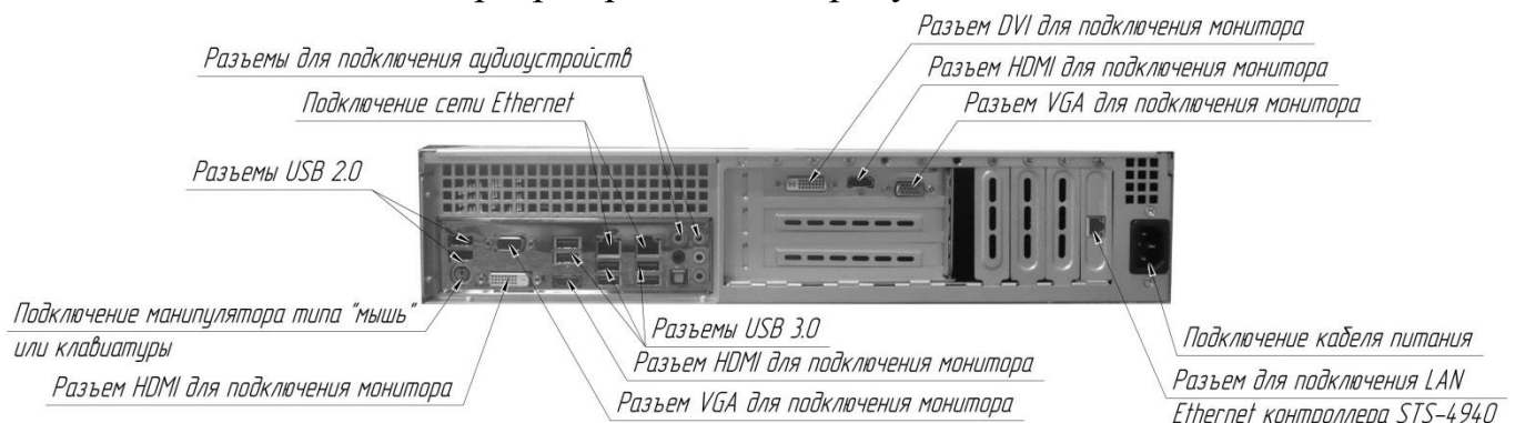
Рисунок 1 – Подключение сервера (расположение, внешний вид и количество разъемов может отличаться от приведенного)
