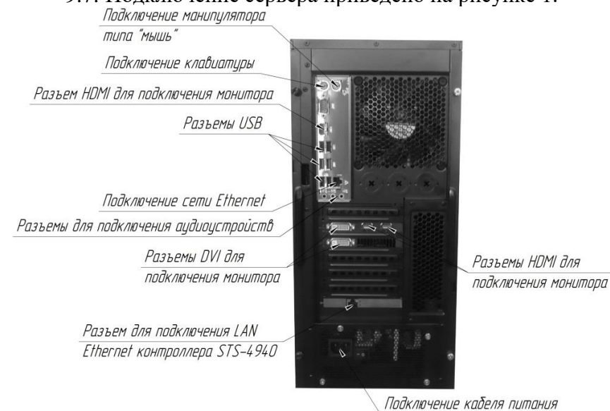
Рисунок 1 – Подключение сервера (внешний вид и расположение разъемов может отличаться от приведенного)
