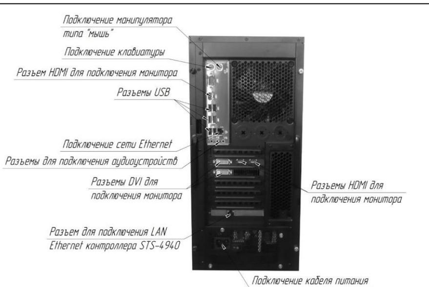
Рисунок 1 – Подключение сервера (внешний вид может отличаться от приведенного)
