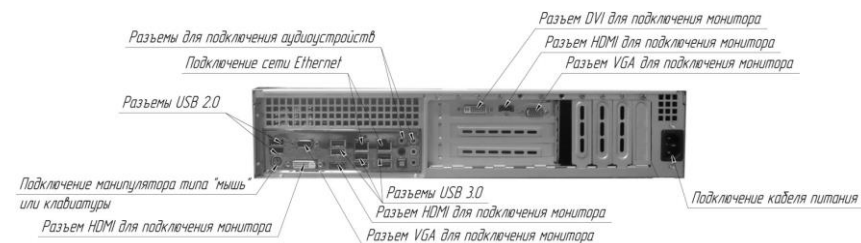
Рисунок 1 – Подключение системного блока (расположение и внешний вид разъемов может отличаться от приведенного)
