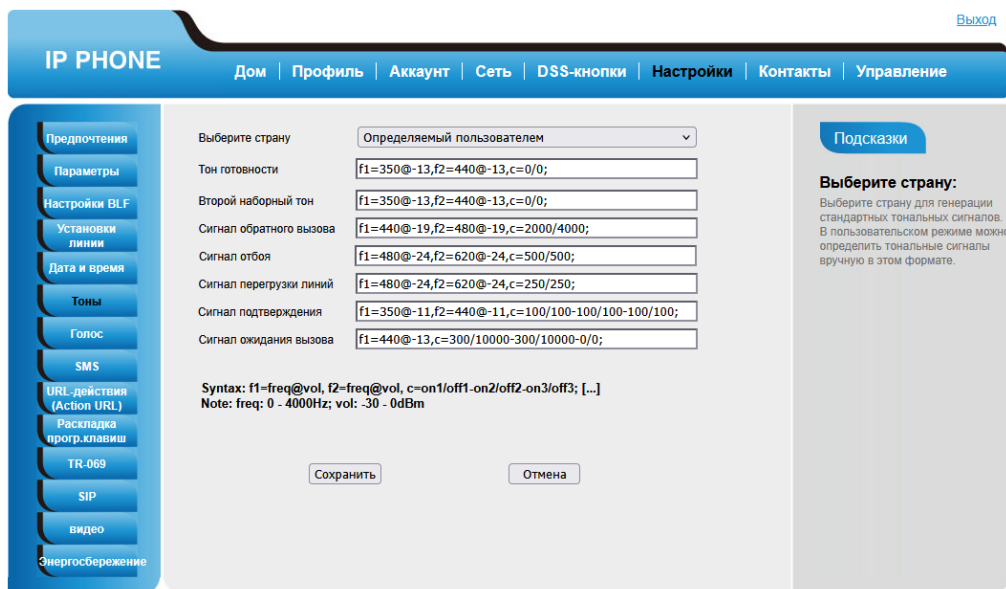
Рисунок 2.26 – Раздел «Тоны»
