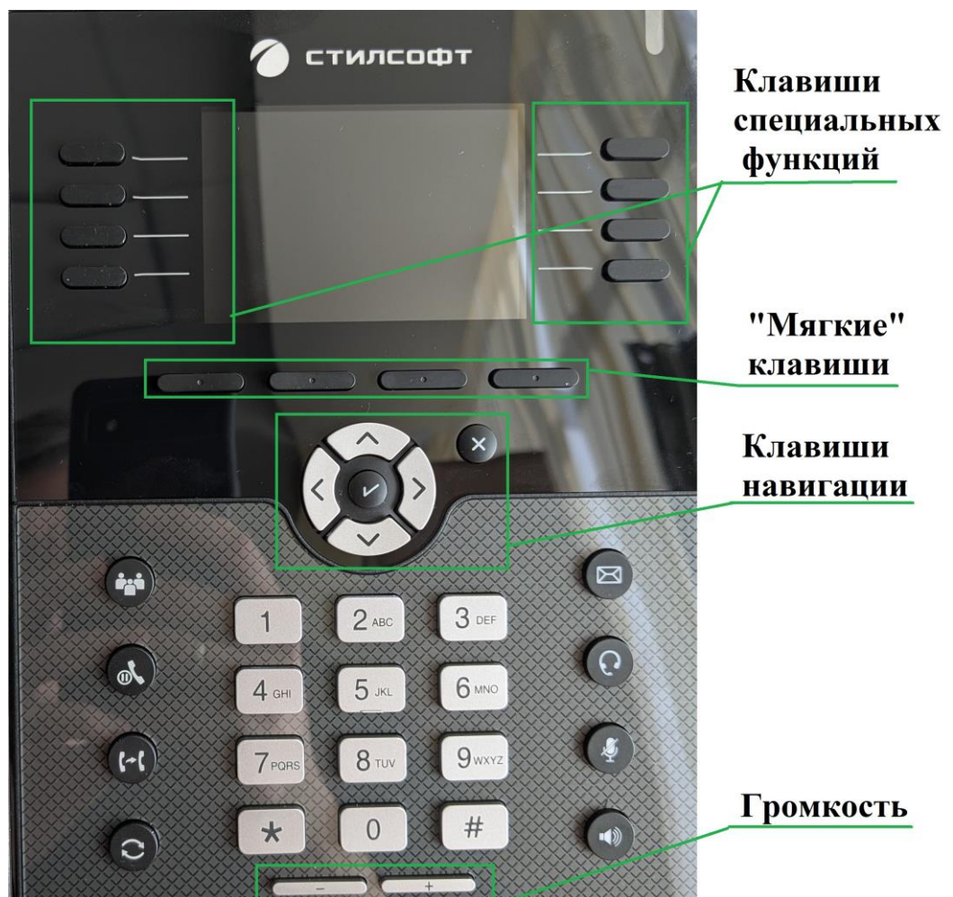
Рисунок 1.2 – Лицевая часть IP телефона STI–101
