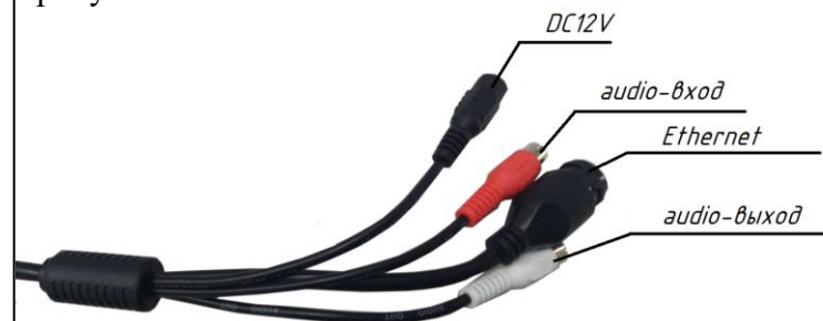
Рисунок 1 – Подключение IP-видеокамеры
