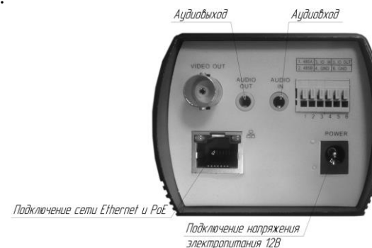
Рисунок 1 – Подключение IP-видеокамеры
